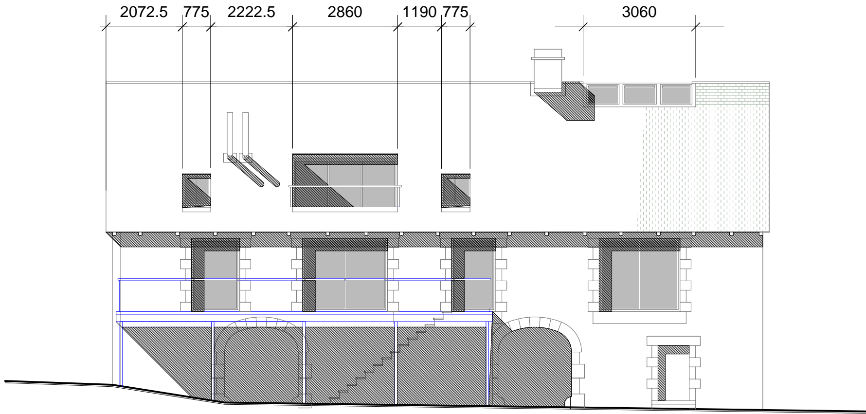
Arriere Elevation
